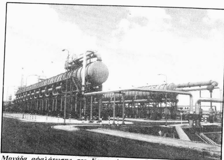
Μονάδα αφαλάτωσης στο Κουρασάο των Ολλανδικών Αντιλλών. Εγκατεστάθη το 1990 και παράγει 10.000 κυβ. την ημέρα!
