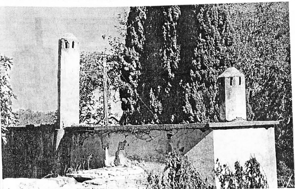
Εικ. 28: Μυλοπόταμος: Νερόμυλος Δημητράκοπουλου. Στο αριό, που εικονίζεται με τις δυο ζαπτιδόχες, υπήρχε η κατοικία του μύλωνά, ενώ σε πρώτο πλάνο φαίνεται καθαρά και το μυλωνάσιο πλάτους 70 εκ.
