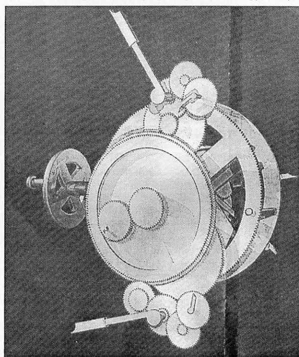
Η πολυπλοκότητα των 30 και πλέον γραναζιών (όπως φαίνεται στο μοντέλο) που κινούσαν τους δείκτες των καντράν του Μηχανισμού καταδεικνύει τη θαυμαστή τεχνολογική πρόοδο των Ελληνιστικών χρόνων.
