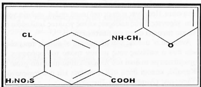
Ο χημικός τύπος της Φουροσεμίδης Elasis
