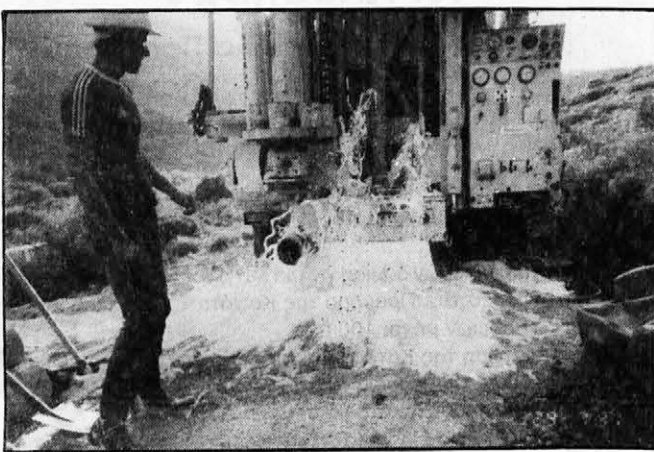
Από την Γεώτρηση της Κοινότητας Μητάων στην Παληόπολη . Η γεώτρηση αυτή απέδωσε 30 κυβ. την ώρα για την ύδρευση Παληόπολης - Αυλέμονα (φωτογρ. Αντων. Πρωτοψάλτη).
