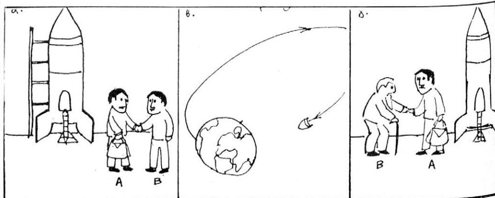
Τρία χρόνια ταξιδιού για τον Α ισοδυναμούν με 30 χρόνια του Β που μένει στη Γη. ΣΧΗΜΑ II.
